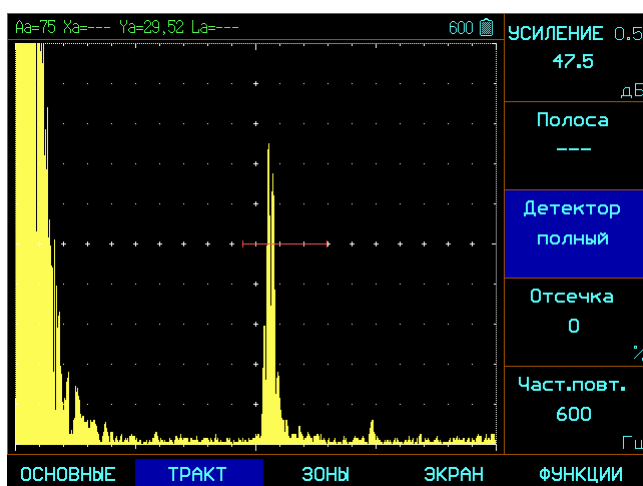
Рис.2-8 Полное детектирование
